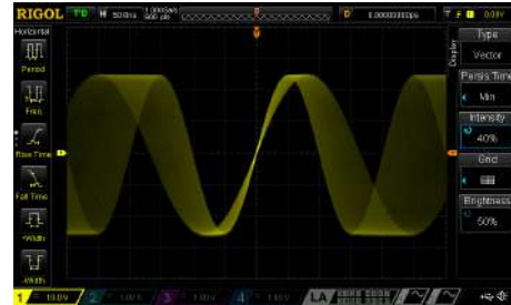
Varias funciones de disparo
