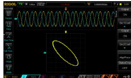
Fuente de 25 MHz de doble canal integrada (DS1XX4Z-S Plus)
