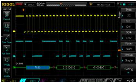
Funciones de decodificador y activador de bus serie (RS232/UART, I2C, SPI)
